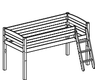
Halbhohes Bett + schräger Leiter L: 210 x T: 136 x H: 118 cm
